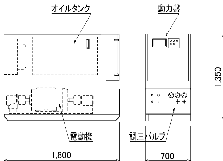
〈油圧ユニット図〉
