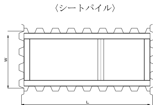
【シートパイル】
