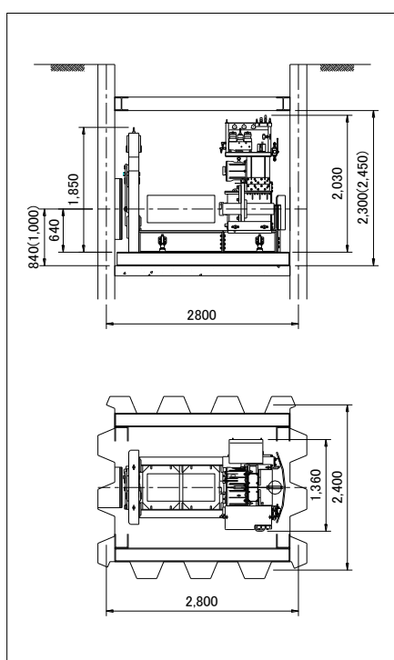
【シートパイル立坑】 (幅 2,400×長 2,800 程度)
