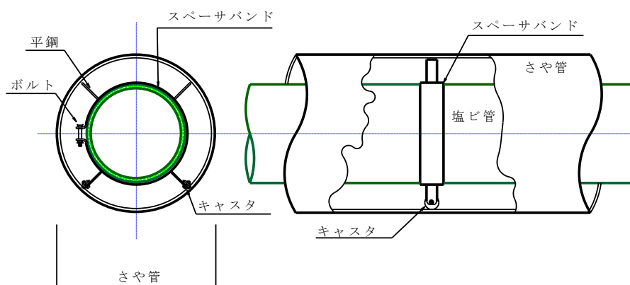
スペーサ設置概念図
