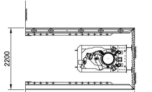
C-C 断面図
