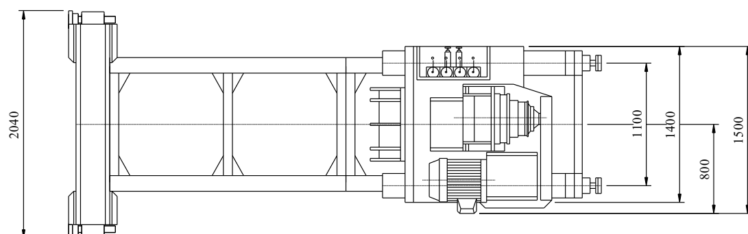
〈本体平面図〉
