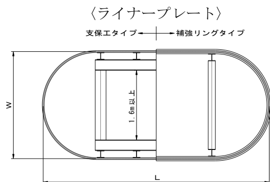
【ライナープレート】
