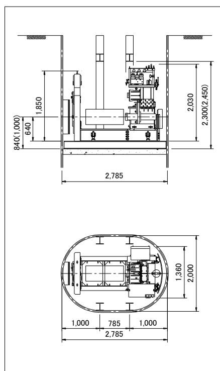
【小判形ライナープレート立坑】 (2,000×2,785)
