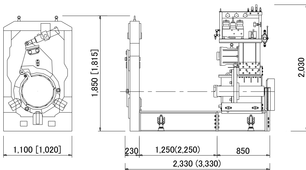
〈本体側面図〉
