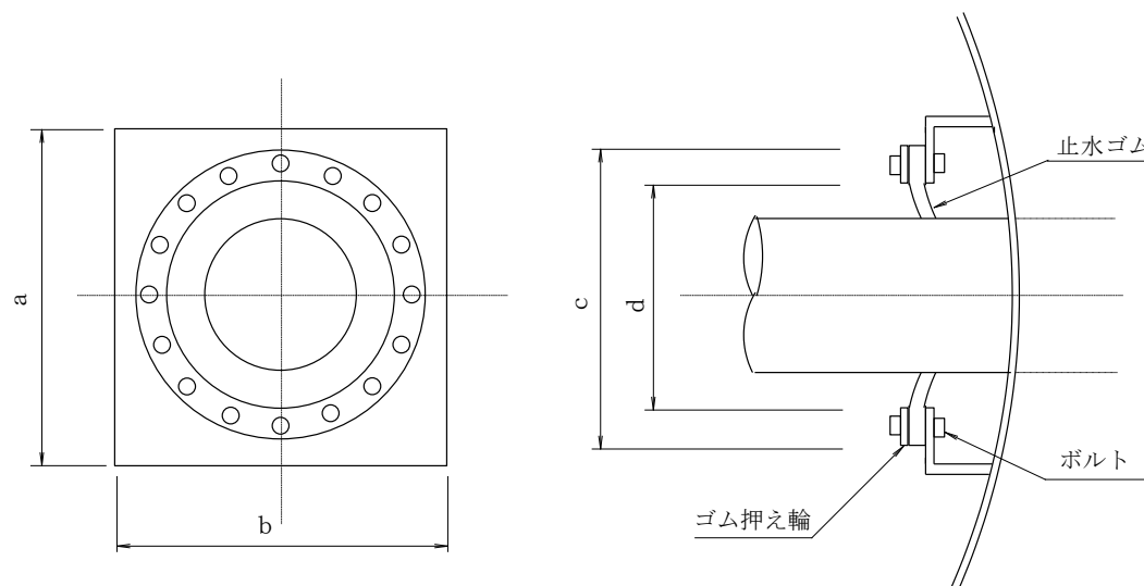
参考図 坑口止水器
